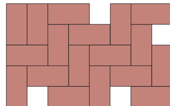
3 BSV-Betontegel elleboog 150x300x80 mm
