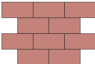
5 BSV-Dubbel-dubbel klinker halfsteens 420x210x80 mm
